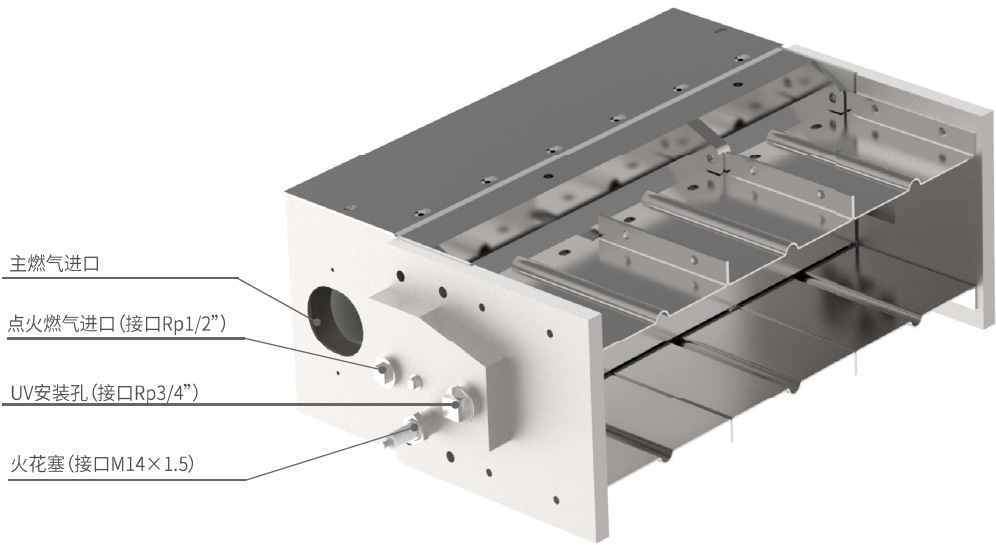
安装示意图
